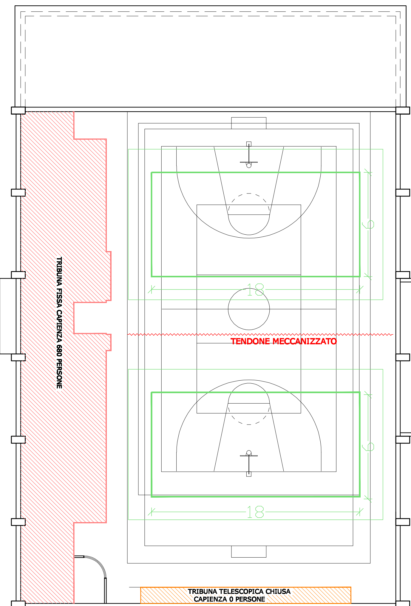
ASSETTO ALLENAMENTI PALLAVOLO (SCALA 1:200)
