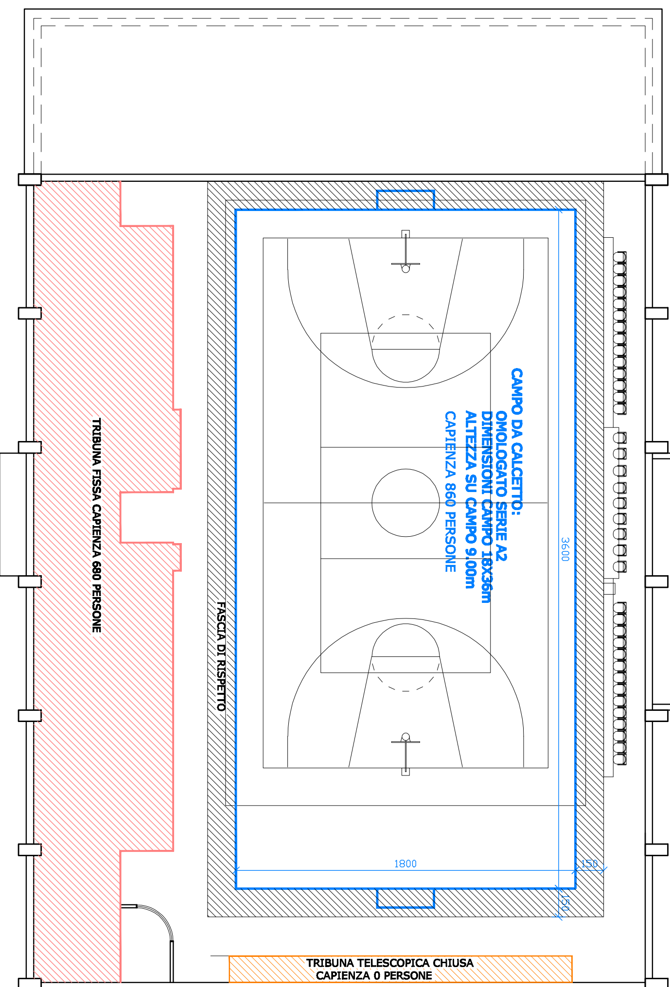
ASSETTO ALLENAMENTI E COMPETIZIONI CALCETTO (SCALA 1:200)
