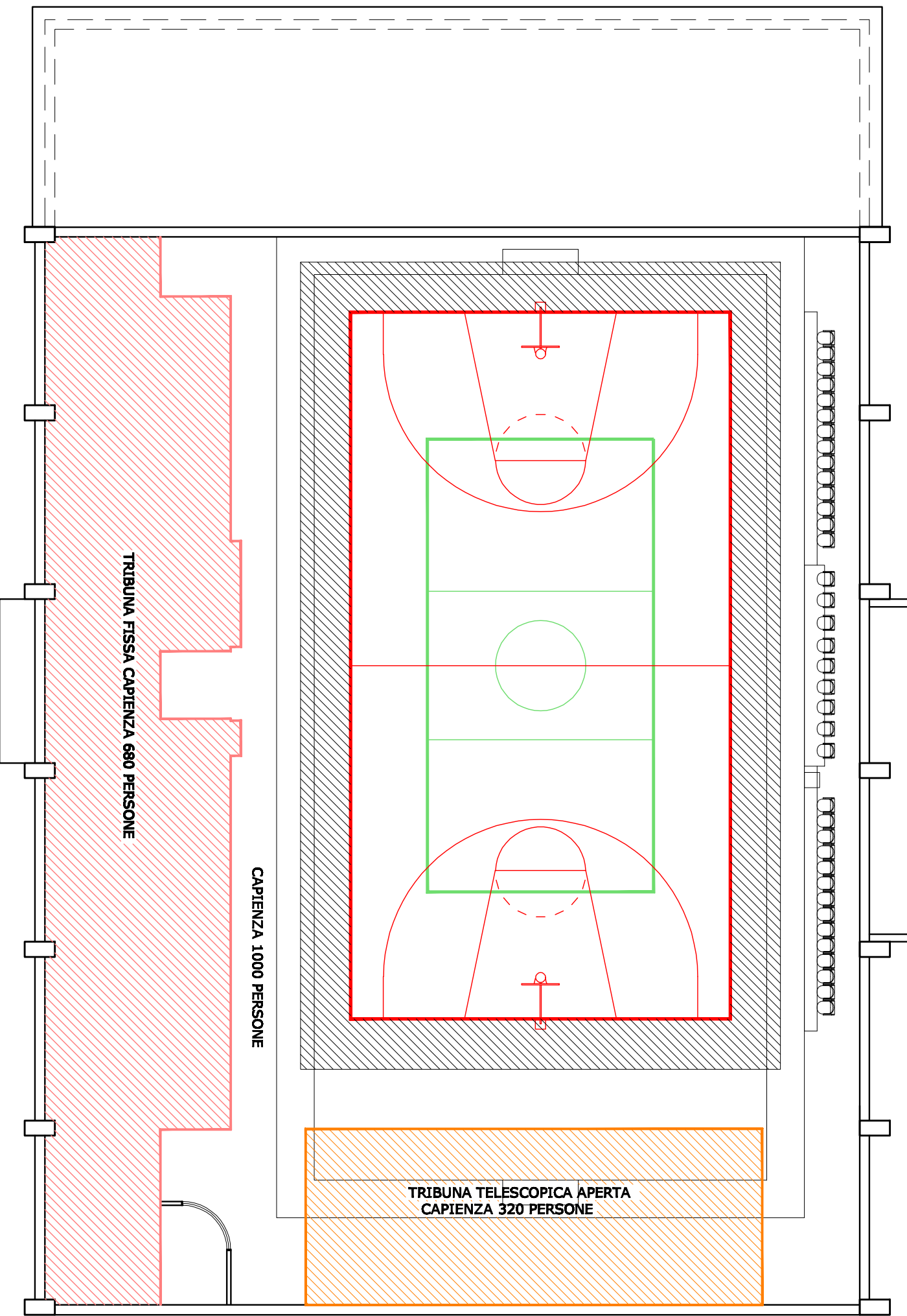
ASSETTO COMPETIZIONI PALLAVOLO E PALLACANESTRO (SCALA 1:200)
